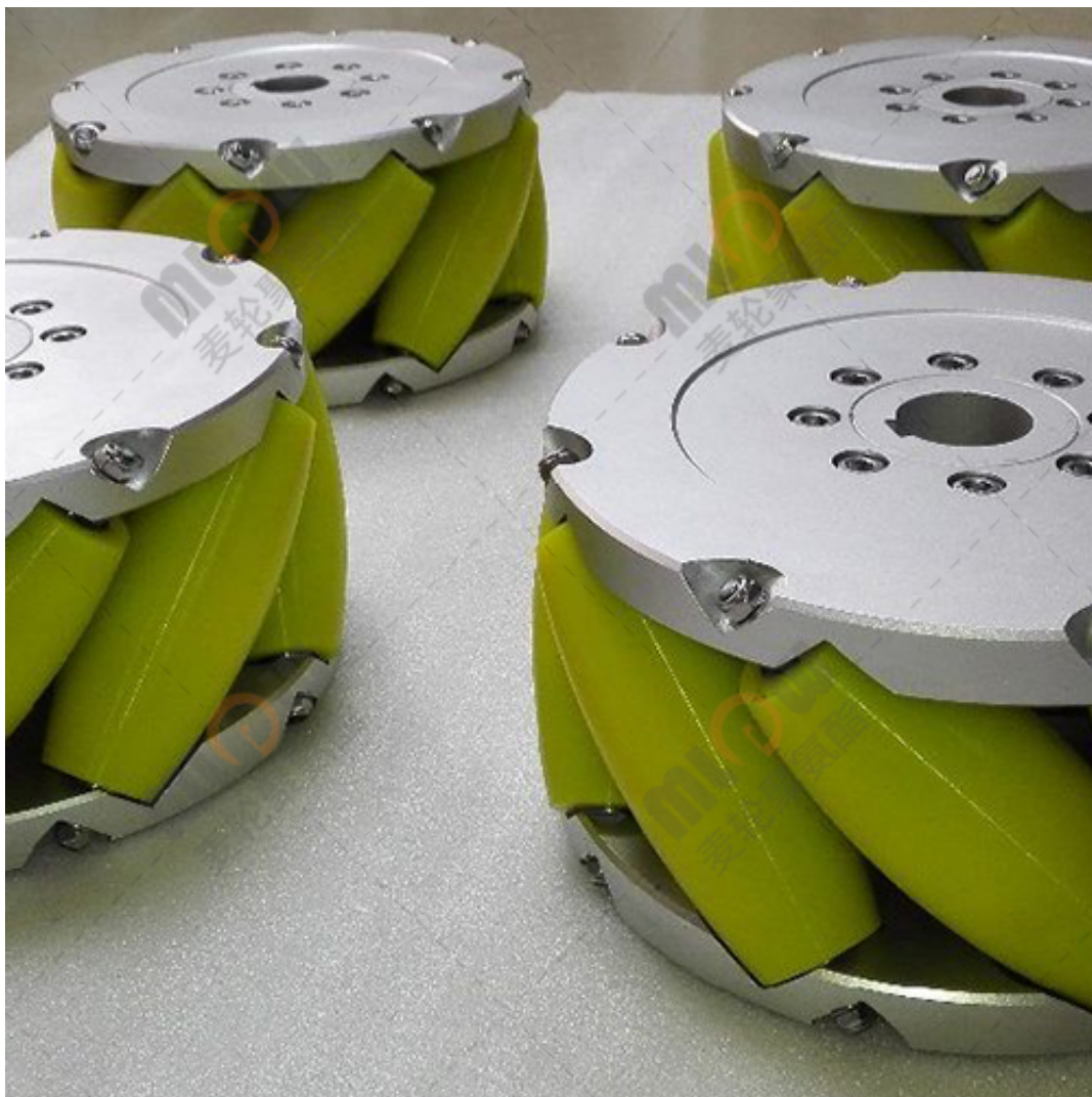
麦克纳姆轮
